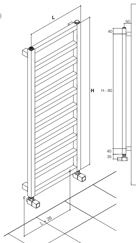
Valvola e detentore "Leo" (26x26 mm) "Leo" valve and lockshield
